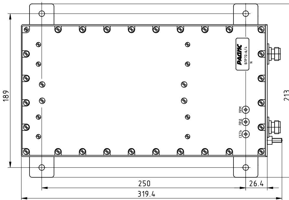
Конвертор БПР70-6/4 внешнего исполнения
