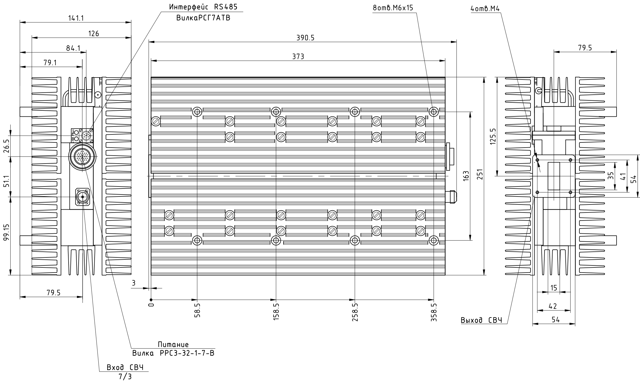
Блок усилителя мощности С-диапазона УМ5964-70 (УМ5765-70)
