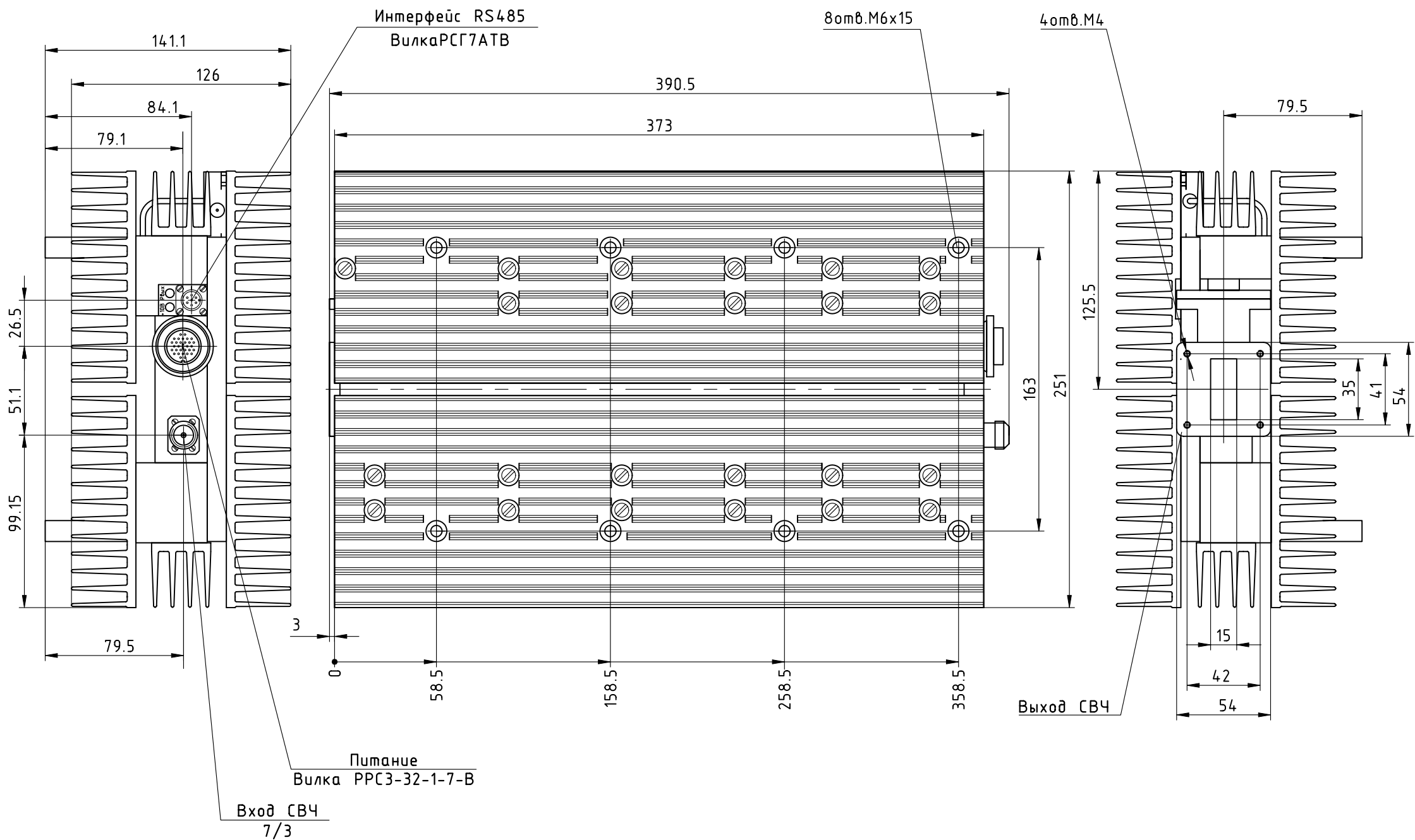
Блок усилителя мощности С-диапазона УМ5964-50 (УМ5765-50)
