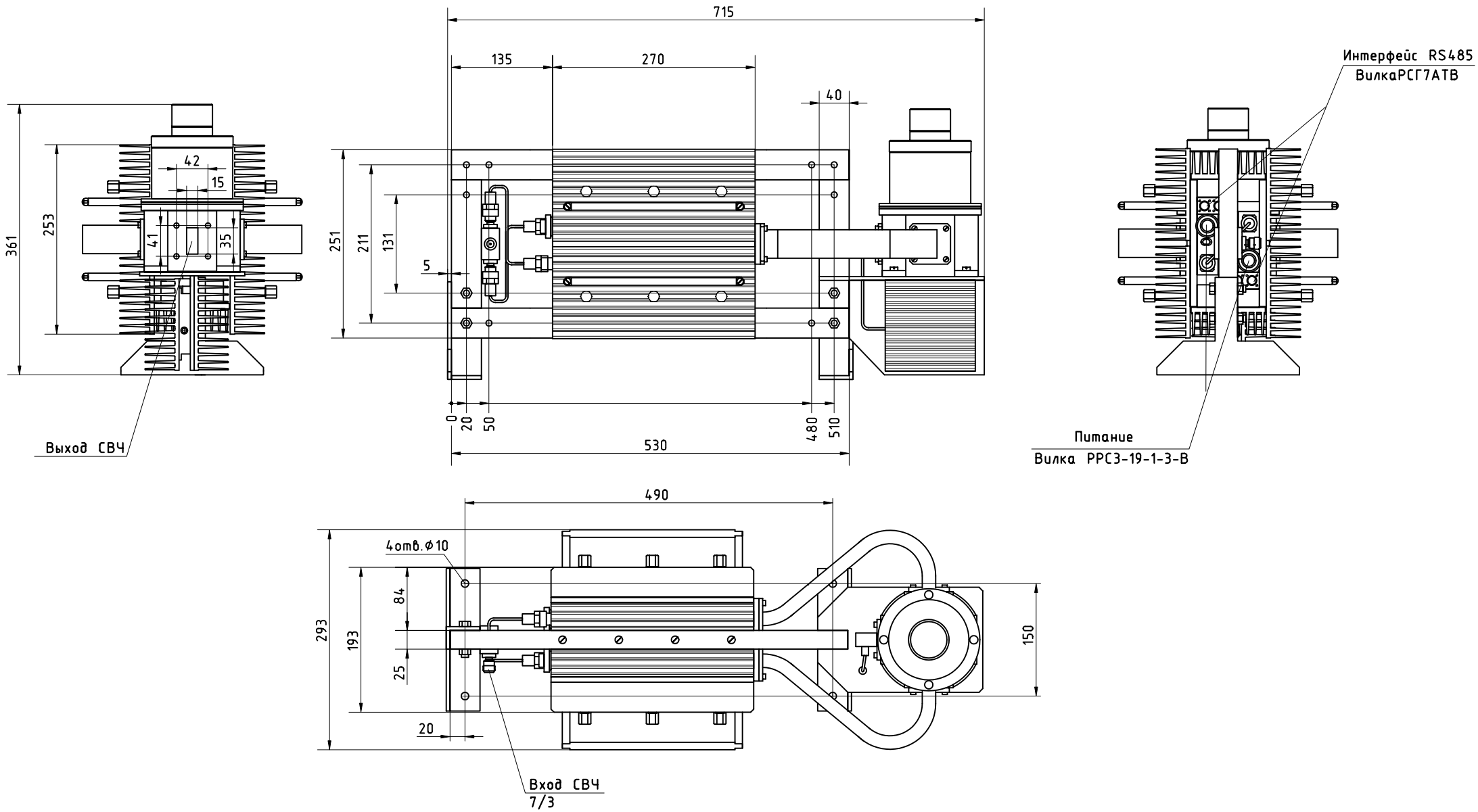
Блок резервированного усилителя мощности С-диапазона УМ5964-25Р (УМ5765-25Р)
