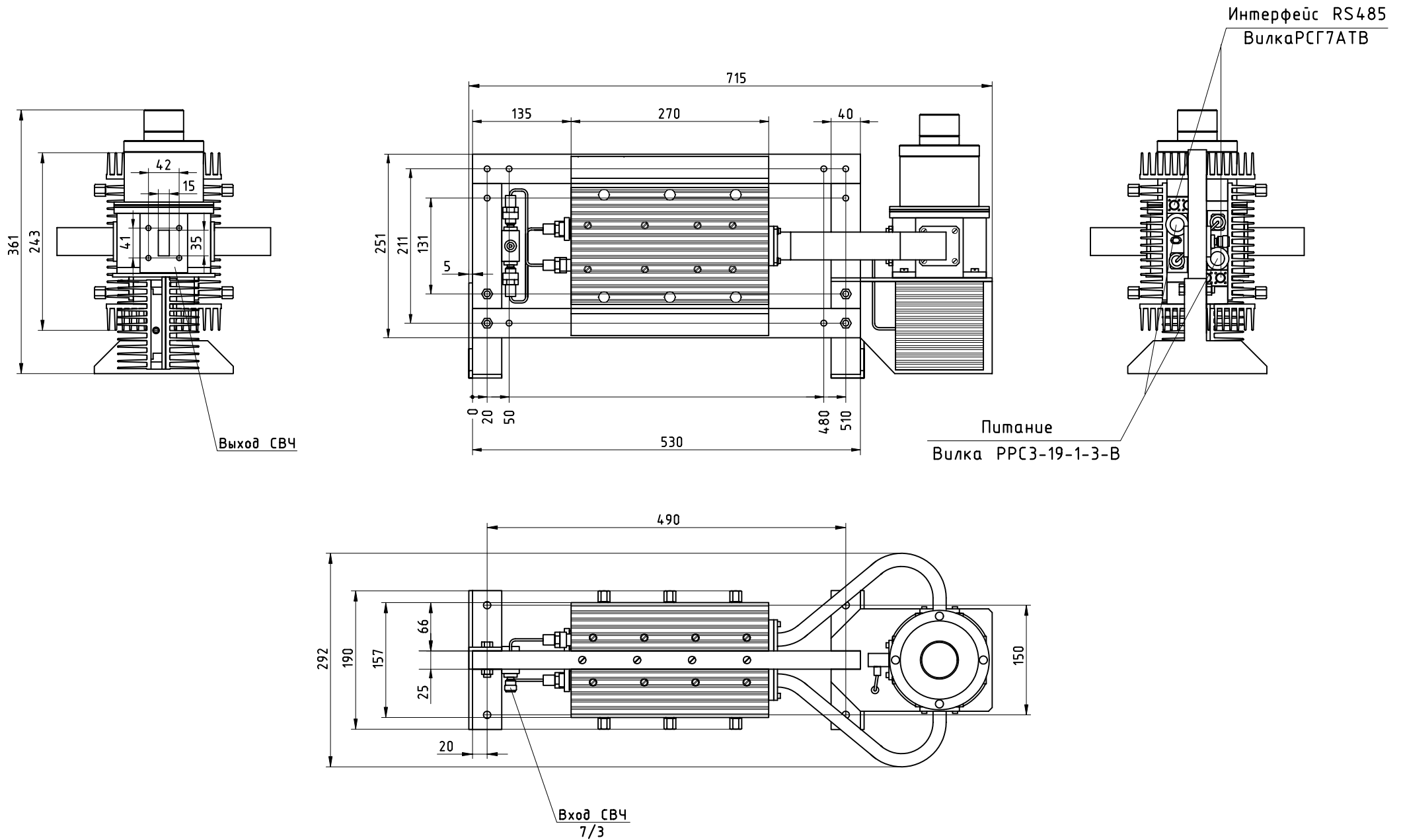
Блок резервированного усилителя мощности С-диапазона УМ5964-15Р (УМ5765-15Р)
